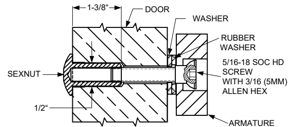
FIG. 2B SOLID DOOR
